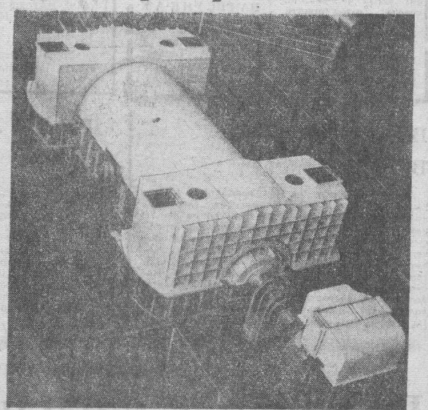
НА ХАРЬКОВСКОМ заводе «Электротражмаш» имени В. И. Ленина (Украинская ССР) изготовлен турбогенератор мощностью 1 миллион киловатт. Он предназначен для испытания своих сверхмощных собратей. У энергогиганта ряд конструктивных особенностей. Так, например, обмотки статора и ротора имеют внутреннее водяное охлаждение, что для подобных генераторов осуществляется впервые. В настоящее время конструкторы завода «Электротражмаш» разрабатывают новые турбогенераторы мощностью до двух миллионов киловатт. НА СНИМКЕ: турбогенератор мощностью 1 миллион киловатт на испытательном стенде завода «Электротражмаш». Фото В. Русинюкского. (АПН).
