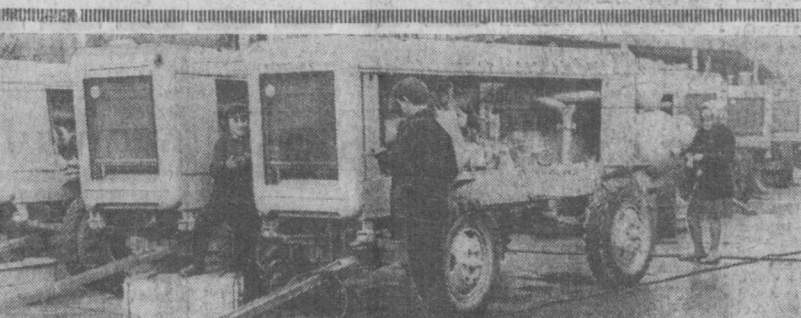
На заводе «Компрессор», как и на других предприятиях города, все шире развешивается соревнование за досрочное выполнение задания девятой пятилетки. НА СНИМКЕ: идет сборка машин в главном сборочном цехе завода. Фото М. Нуриддинова.
