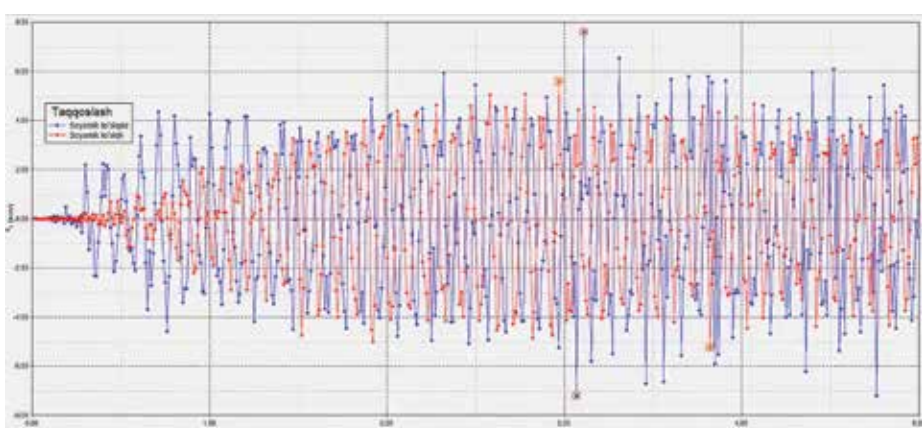
7-rasm. 32-kuzatuv nuqtasidagi tezlanishni taqqoslash grafigi.
