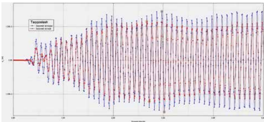
5-rasm. 32-kuzatuv nuqtasidagi ko'chishni taqqoslash grafigi, mm.
