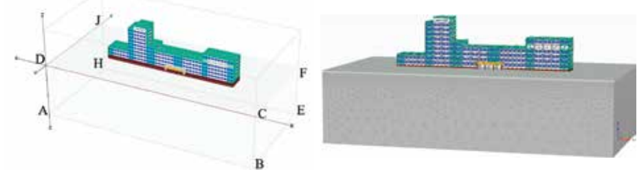
1-rasm. Plaxis 3D dasturida modelashtirish va chekli elementlarga bo'lish jarayoni.
