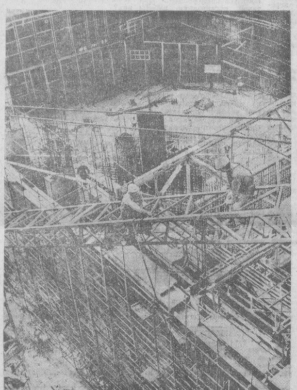
Строительство первой в Болгарии атомной электростанции в Козлодуме отмечено важным событием — началом возведения бетонных стен первого реакторного отделения, где разместится один из реакторов станции мощностью 440 тысяч киловатт. Всего в Козлодуме будет установлено два таких реактора.
