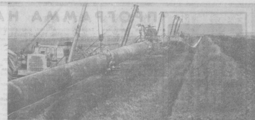
Специалисты объединения «Уралмаш» участвуют в наладке и пуске сложных установок на металлургических предприятиях братских стран. НА СНИМКЕ слева: монтаж дробилки, предназначенной для отправки в ПНР. В Хмельницкой области проходит один из наиболее сложных участков газопровода Оренбург — Западная граница СССР, строительство которого осуществляется в рамках СЗВ. В работах принимает участие специалист из Венгерской Народной Республики. НА СНИМКЕ: укладка труб на территории Дунаевского района.
