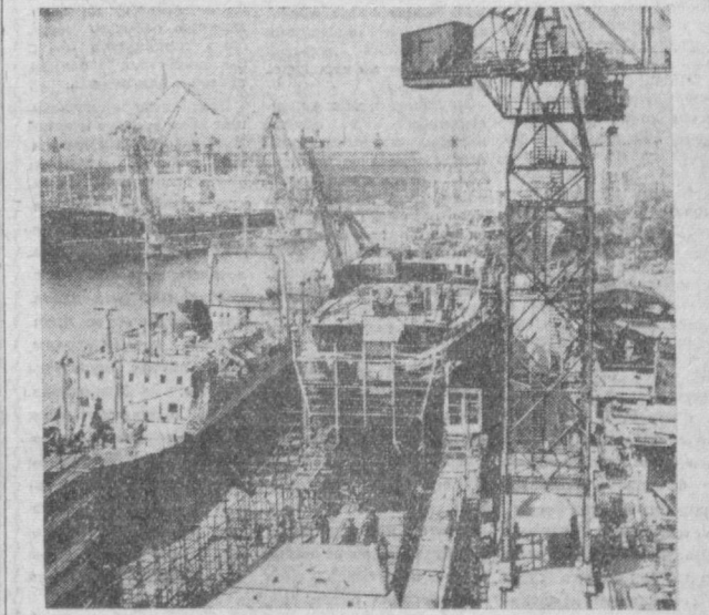
Судоостроительная промышленность Польши — одна из новых отраслей индустрии, созданной за годы народной власти. Судоостроительная верфь в Гданьске, в прошлом строившая небольшие рыбачьи катера и лодки, сейчас выпускает продукцию на уровне современного мирового судостроения. За 20 лет со стальной верфи сошло более 520 судов, из которых 400 построено по заказу Советского Союза. Крупные грузовые суда, современные траулеры строятся на верфи имени Пармиской Коммуны в Гданьке и верфи имени А. Варского в Щецине.
