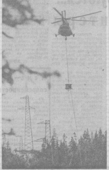
ВЕРТОЛЕТ-МОНТАЖНИК ЛЭП
