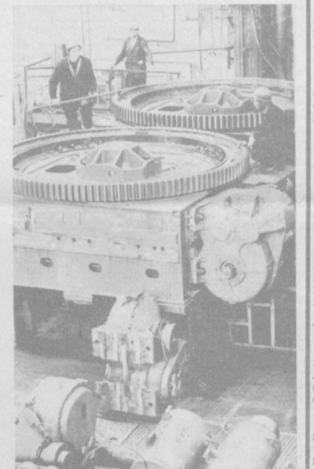
НА СНИМКЕ: сборка деталей пятнубовых экскаваторов для стран — членов СЭВ.
