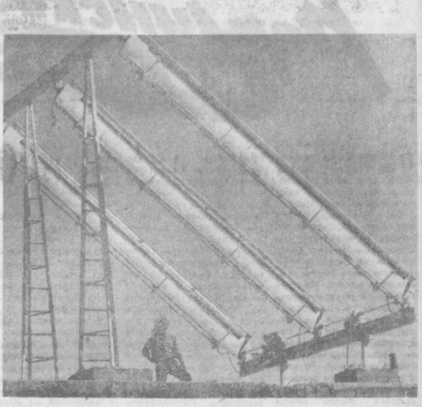
НА СНИМКАХ: справа — это солнечная электростанция опреснителя. Она состоит из отдельных фотоэлементов, преобразующих лучистую энергию солнца в электрическую. Мощность станции 500 ватт. Ее энергия вращает электродвигатели насосов, которые поднимают воду из колодца 12-метровой глубины; внизу — опреснитель (слева), солнечная электростанция и водопойное устройство на пастбище совхоза. Фото С. Корытникова.
