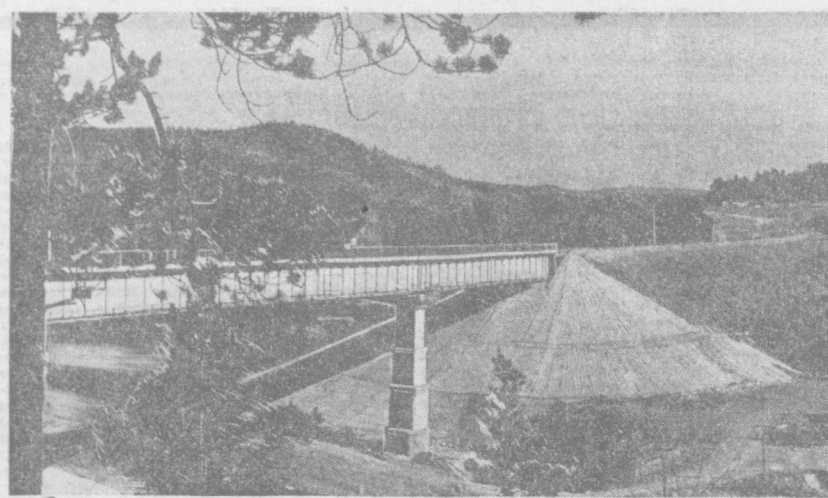
БАШКИРСКАЯ ЖЕЛЕЗНО-ДОРОЖНАЯ СТАНЦИЯ. На строительстве железной дороги Белоречье — Чимши заканчивается укладка пути на участке Белоречье — Инзер, длиной 82 км. Скоро железная дорога придет в поселок Инзер. На станции с одноименным названием будут доставлены материалы для строительства вокзала, локомотивного депо, жилья.
