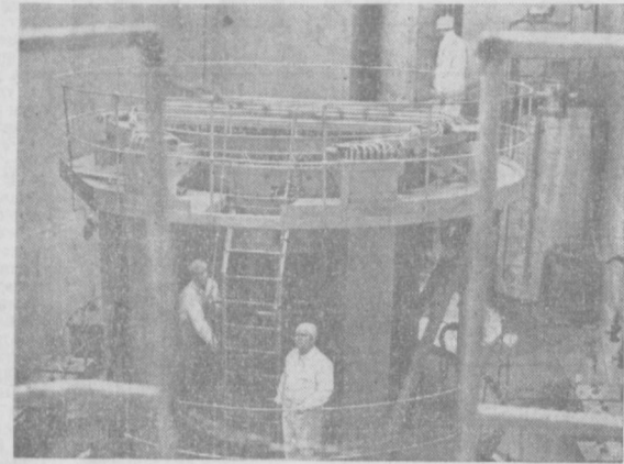
ВОРОНЕЖ, НА НОВОВОРОНЕЖСКОЙ АТОМНОЙ ЭЛЕКТРОСТАНЦИИ ВСТУПИЛ В СТРОЙ ВТОРОЙ ЭНЕРГБЛОК МОЩНОСТЬЮ 375 ТЫСЯЧ КИЛОВАТТ, ПОЛУЧЕНЫ ПЕРВЫЕ КИЛОВАТТ-ЧАСЫ ЭЛЕКТРОЭНЕРГИИ.
