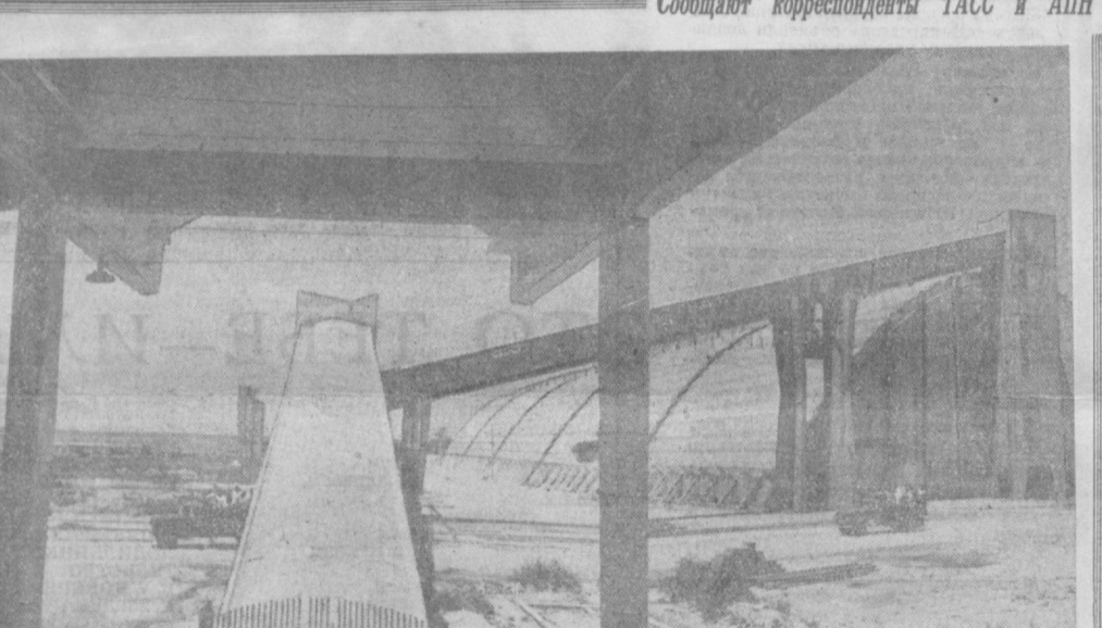
В послереволюционные годы на Кубе началась борьба за ускорение погрузки сахара в суда и экономии при этом средств. С этой целью в трех портах страны — Матансаса, Сьенфуэгосе и Гуабиале — построены специальные поточные линии и хранилища. Эти сооружения позволили избежать стране на погрузке сахара расходы в размере 10 миллионов долларов. В результате практически отпала необходимость в мешках, а также почти в десять раз ускорилась обработка судов, получающих на Кубе сахар. НА СНИМКЕ: общий вид поточной линии и сахарохранилища в Сьенфуэгосе. Фото С. Преображенского.
