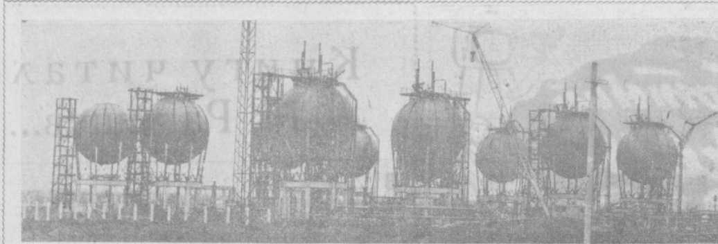
На окраине Грозного заканчивается монтаж крупнейшего на Северном Кавказе парка шаровых резервуаров для хранения нефтепродуктов под давлением. Емкости смонтированы монтажными Грозненского специализированного управления ордена Ленина треста М 7.
