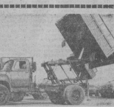
КИРГИЗСКАЯ ССР. Недавно с конвейера Фрунзенского автозавода сошла новая модель самосвала. Платформа машины может не только откидываться на три стороны, но и подниматься на высоту до двух метров. НА СНИМКЕ: новая модель самосвала. Фото В. Утешева. (Фотохроника ТАСС).
