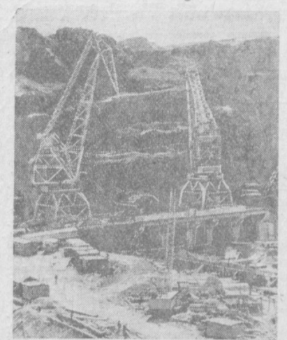
Вид строительства Капчагайской ГЭС, сооружаемой недалеко от Алма-Аты на реке Или. Фото Б. Клипницера. (Фотокхроника ТАСС).
