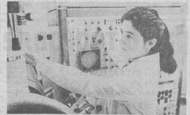
Весомый вклад в расширение минерально-сырьевой базы действующих и строящихся предприятий республики, в открытие месторождений и подготовку их к эксплуатации вносит Институт геологии и геофизики АН УзССР. В исследовании минералов геологам помогает современная электронная техника. НА СНИМКЕ: старший инженер кабинета физических методов М. Мусева ведет подготовку микрозона к анализам. Фото М. Нуриддинова.
