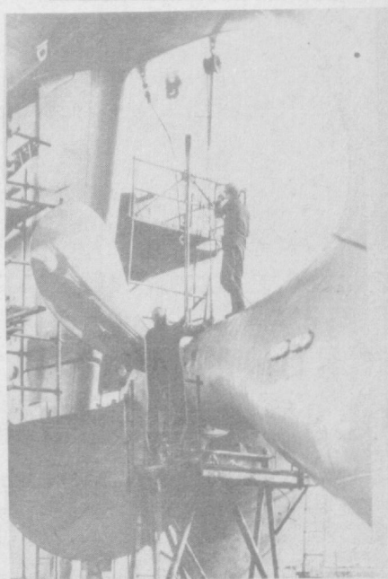
Строительство контейнеровозов типа «Меркур-2» — 174-метровых гигантов, берущих на борт до 940 контейнеров, — осуществляется на одной из крупнейших в ГДР ростокской верфи «Варнов-верфт». В этом году корабельщики передадут советским заказчикам еще три таких мощных грузовых судна новой серии. НА СНИМКЕ: на монтаже гребного винта очередного строящегося контейнеровоза. Фото АДН-ТАСС.
