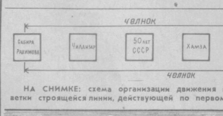
НА СНИМКЕ: схема организации движения поездов Ташкентского метрополитена при производстве работ по строительству соединительной ветки строящейся линии, действующей по первому пути перегона «Пахтакор» — «Дружба народов».
