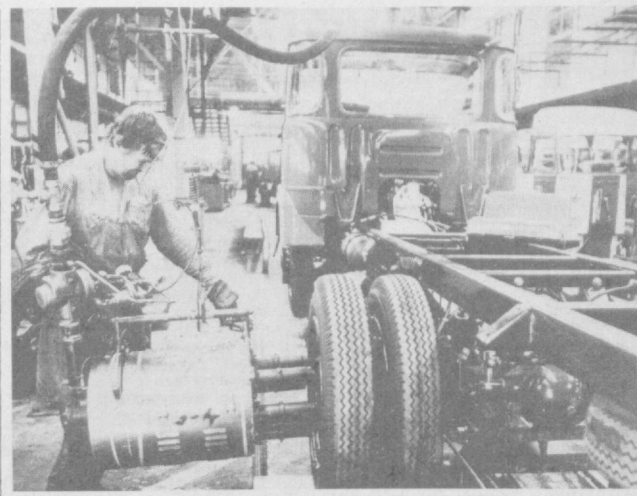
ЧЕХОСЛОВАКИЯ. Высокая экономичность — главная отличительная черта малогабаритных грузовиков и автофургонов, выпускаемых пражским автомобильным заводом «Авиа». В условиях города, при частых остановках, запусках и изменении режима работы двигателя расход дизельного топлива не превышает 13 литров на сто километров. Эти автомашинки имеют большую скорость, маневренность, практически бесшумный двигатель с пониженным выхлопом газов. В этом году столичное предприятие отравило в СССР три тысячи таких машин, что составит почти половину всего заводского экспорта. НА СНИМКЕ: на главном конвейере завода «Авиа». Фото ЧТК—ТАСС.
