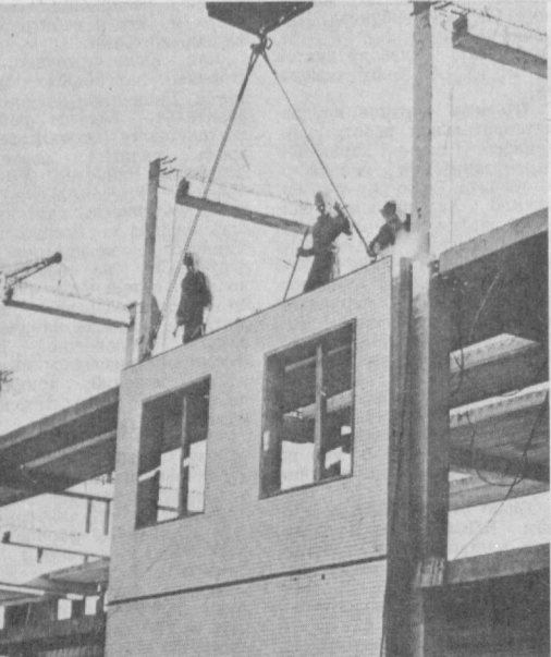
Монтажники Н. Ковалев, В. Малаянц и сварщик С. Монастырский из комплексной бригады А. Янушкевича (СУ-22 треста № 159 Главташкентстроя) ведут монтаж укрупненных наружных стеновых панелей на строительстве школы № 18 на массиве Юнусбад.
