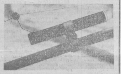
МОСКВА. Этот приборчик — электрический сигнализатор «Светлячок-ЭСП-1», поступающий в продажу, предназначен для рыболовов-любителей. При клеве от натяжения лески замыкается контакт приборчика и загорается лампочка.
