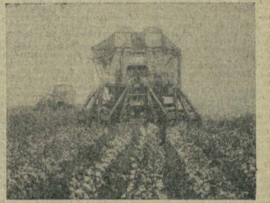
Ташкентской области проходит государственные испытания две шестирядные хлопкоборочные машины «ХВ-54», разработанные и созданные в ГСНБ по машинам для хлопководства под руководством ведущего конструктора Игоря Николаевича Флавицкого.
