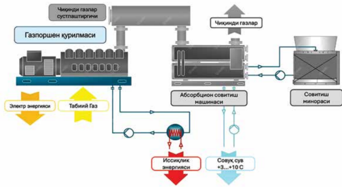
▲ Қурилманинг тузилиши.
