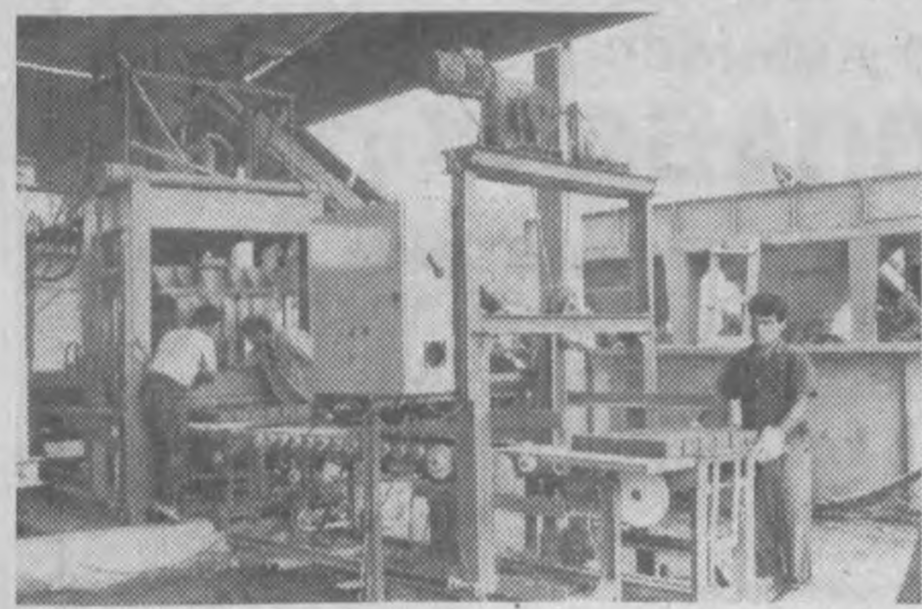
НА СНИМКАХ: на этой площадке сушится кирпич; с помощью этой установки кирпич формируется под высоким атмосферным давлением.
