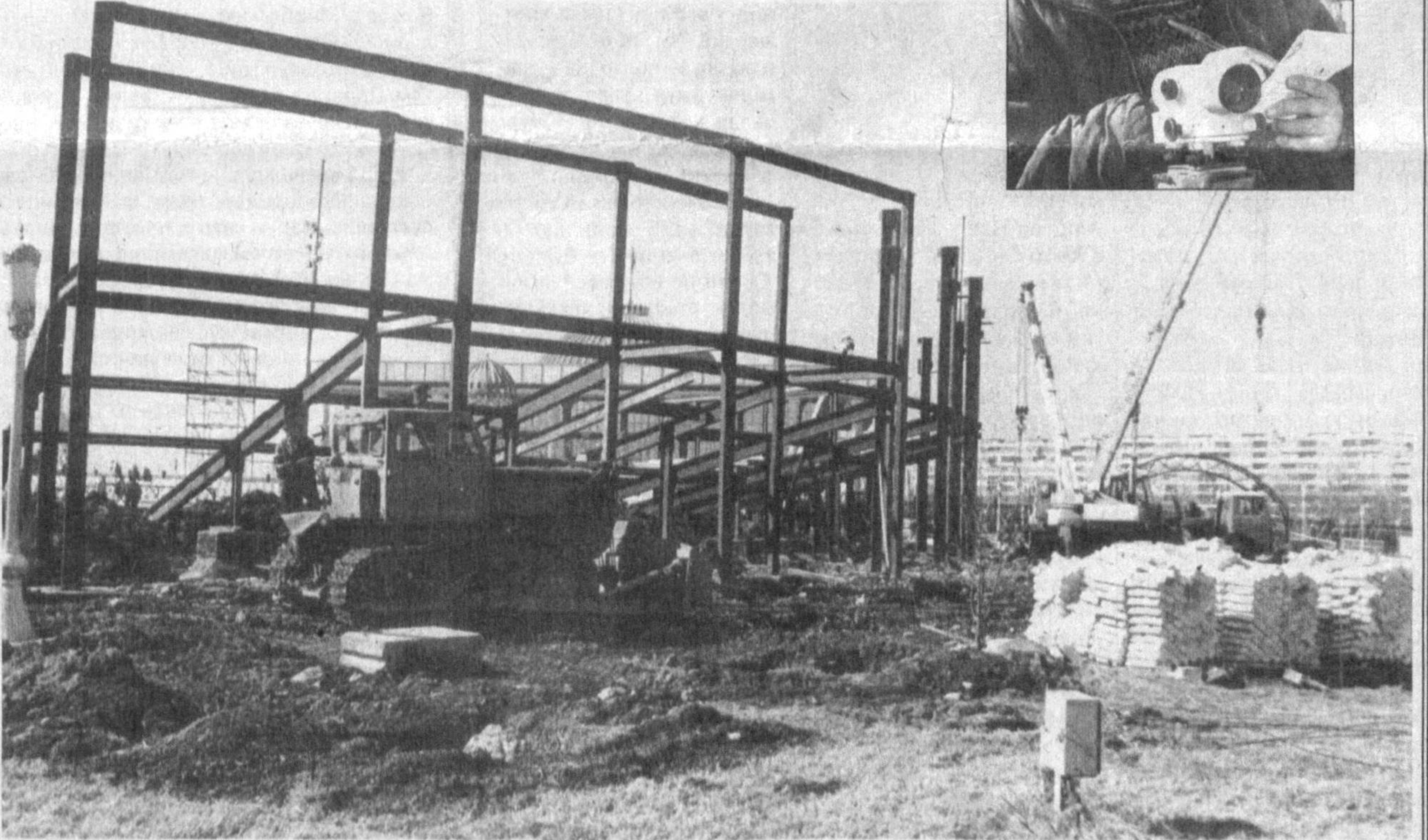
СУРАТЛАРДА: ишбоши Комил Каримов (ўртада) бригадир Зухриддин Акмалов ҳамда тикловчи Шомурод Йўлдошевга кўрсатма бермоқда; геодезчи Абдор Жумаев; қурилиш-тиклаш ишлари давом этмоқда. Сергей Любич олган суратлар.
