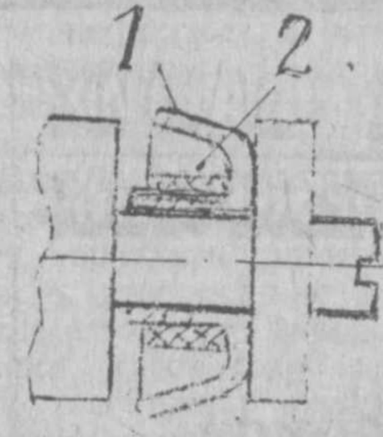
РИС. 1 УПЛОТНЕНИЕ ПОСАДКИ МАНЖЕТЫ-1 ПРИ ПОМОЩИ КОЛЬЦА-2
