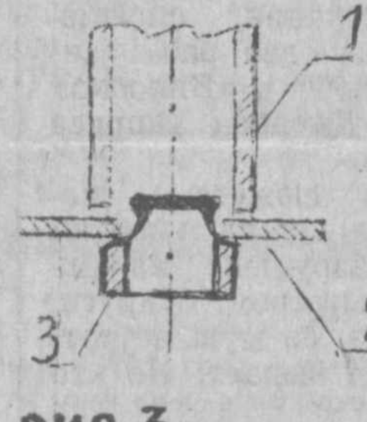
РИС. 3 ЗАПРЕССОВКА КОЛПАЧКА-3 ПРИ ПОМОЩИ ШАЙБЫ-2 И ТРУБКИ-1
