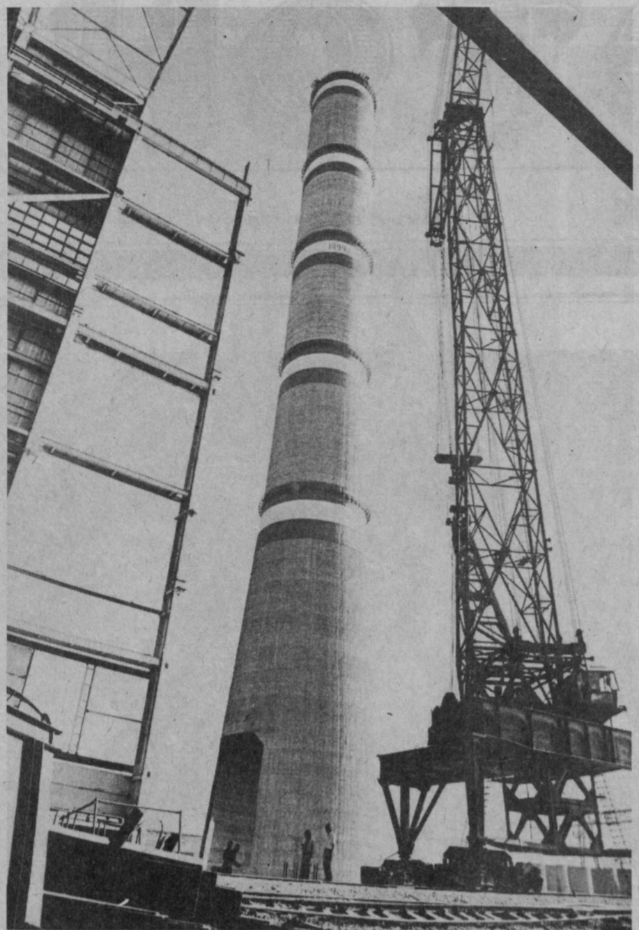
Талимаржон ГРЭСи нафақат Ўзбекистон, балки Марказий Осиё ҳудудда ҳам ўз қуввати, ишлаб чиқариш суръати билан етакчи урилларда туради. Суратдаги тугун қувуриги тиклаш учун 2200 тонна металл ва 11 тонна бетон қоринмаси ишлатилди. Унинг баландлиги 270 метр.
