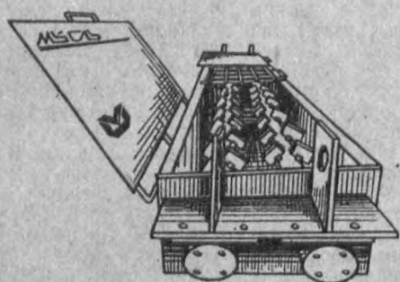
Лой аралаштирувчи икки валли КМ 01 ва КМ 01А ускунаси
