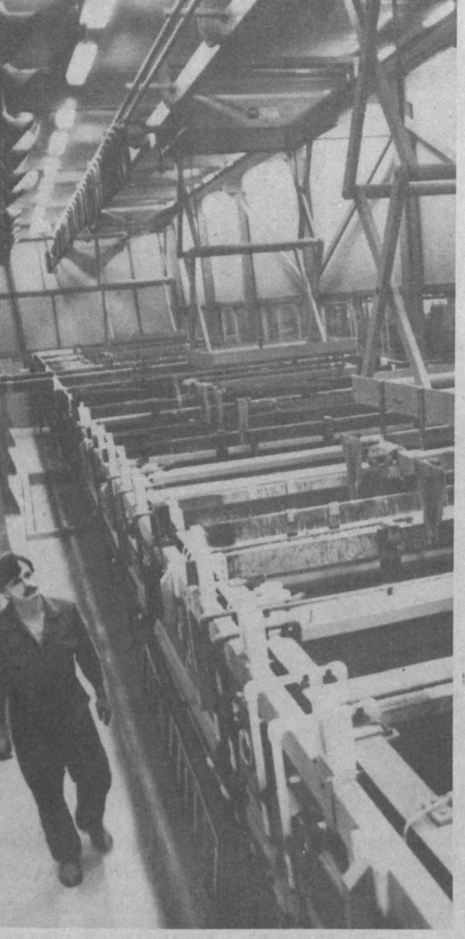
Пуск новой гальванической линии, смонтированной на головном предприятии научно-производственного объединения «Средазэлектроаппарат» шведской фирмой «Гальвоур», позволил полностью ликвидировать вредные выбросы при цинковании деталей электрооборудования, выпускаемого объединением.
