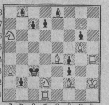
Мат в три хода.
