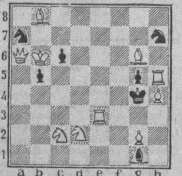
Мат в два хода.
