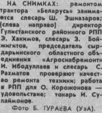
НА СНИМКАХ: ремонт трактора «Беларусь» занимается слесарь Ш. Эшазаров; (слева направо) директор Гулистанского районного РПП Э. Хакимов, слесарь З. Бойжигитов, председатель сирдарьинского областного объединения «Агротехремонт» И. Ибодуллаев и слесарь С. Рахматов проверяют качество ремонта техники; работа в РПП для О. Корожанова — удовольствие; токарь И. Сулаймонов. Фото Б. ТУРАЕВА (УзА).
