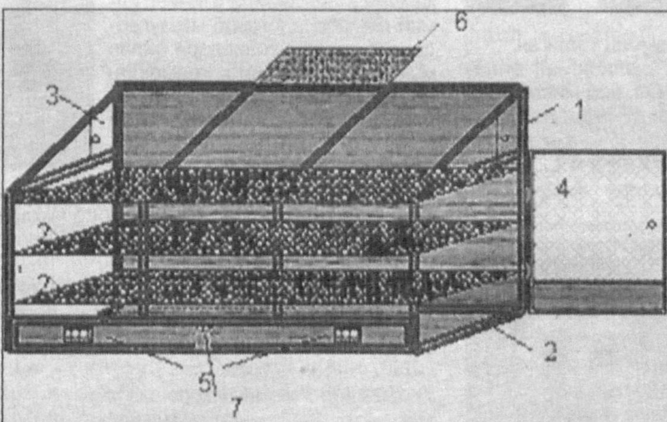
1. Қурилма. 2. Турли стеллажлар. 3 ва 5. Ҳаво алмаштиргич. 4. Шиша эшик. 6. Қуёш батареяси. 7. Вентилятор.
