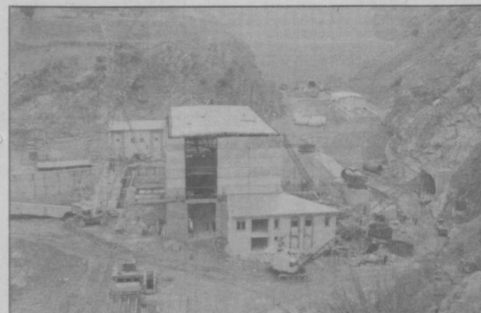
На «ТуполангадГЭСстрое» в эти жаркие майские дни работа ведется в две смены. Идет монтаж гидротурбин и другого оборудования, завезенных из России и Украины.
