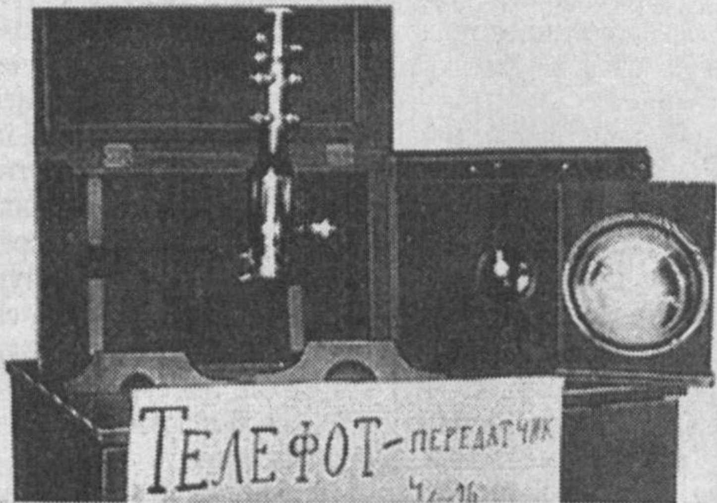
Оптика и передающая трубка телефота, 1926 г.
