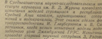
В Среднеазиатском научно-исследовательском институте ирригации им. В. Д. Журина проводятся испытания моделей строящихся в республиках Средней Азии каналов, ирригационных сооружений и водохранилищ. Этот снимок сделал фотокорреспондент И. Глауберзон и В. Сироткин, когда велись испытания модели водозаборного узла Джамбулской ГРЭС. Испытание проводит старший научный сотрудник З. Радова и старший техник М. Великанов.
