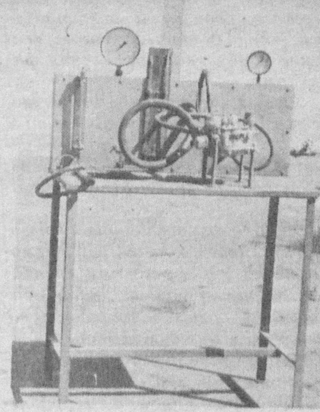
Стенд для контроля параметров газовых редукторов
