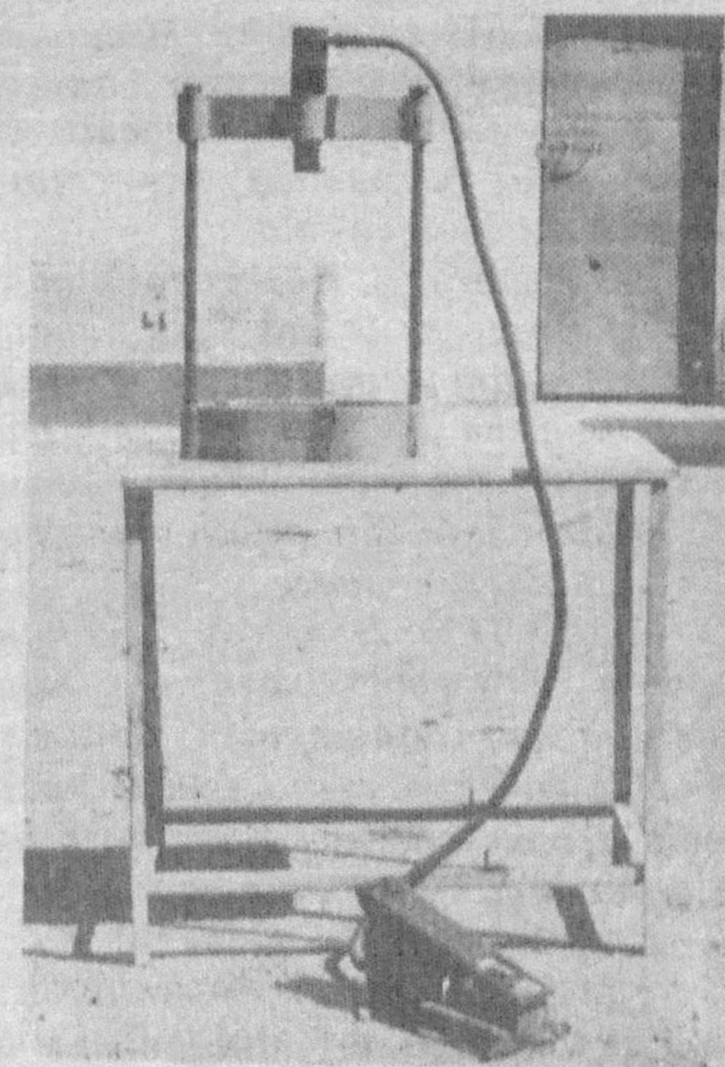
Пресс гидравлический
