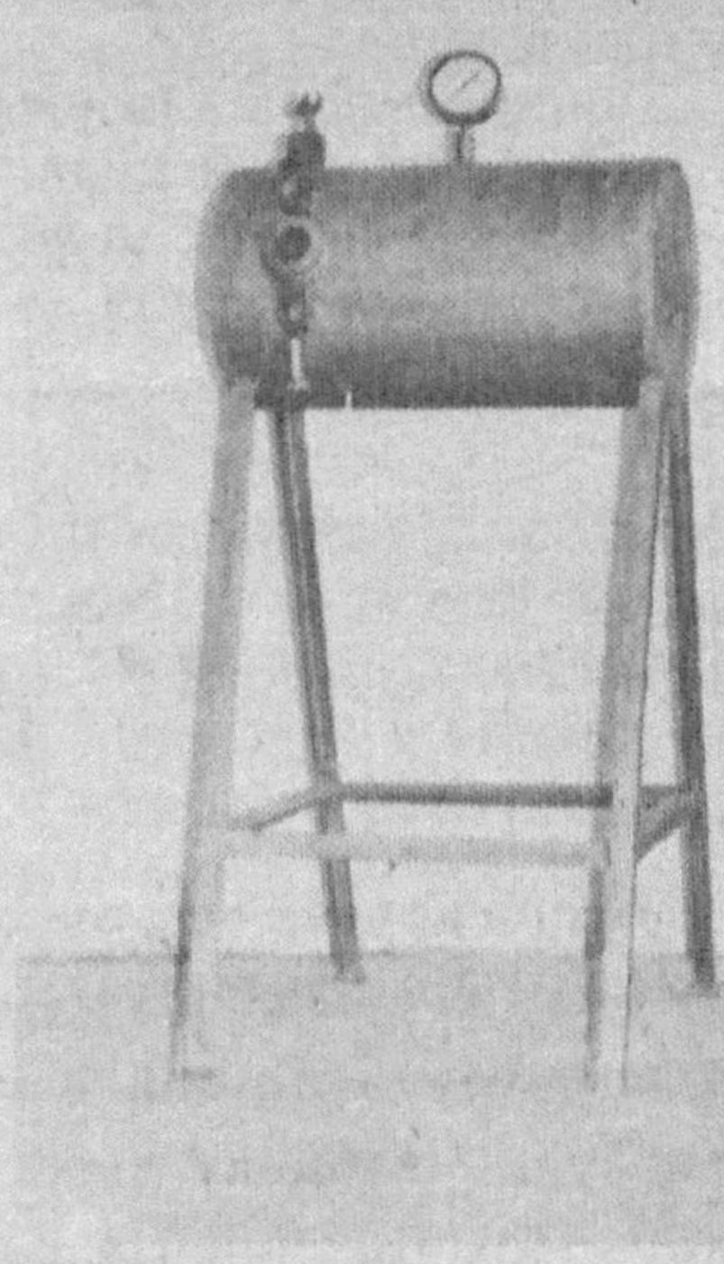
Стенд для проверки блока арматуры
