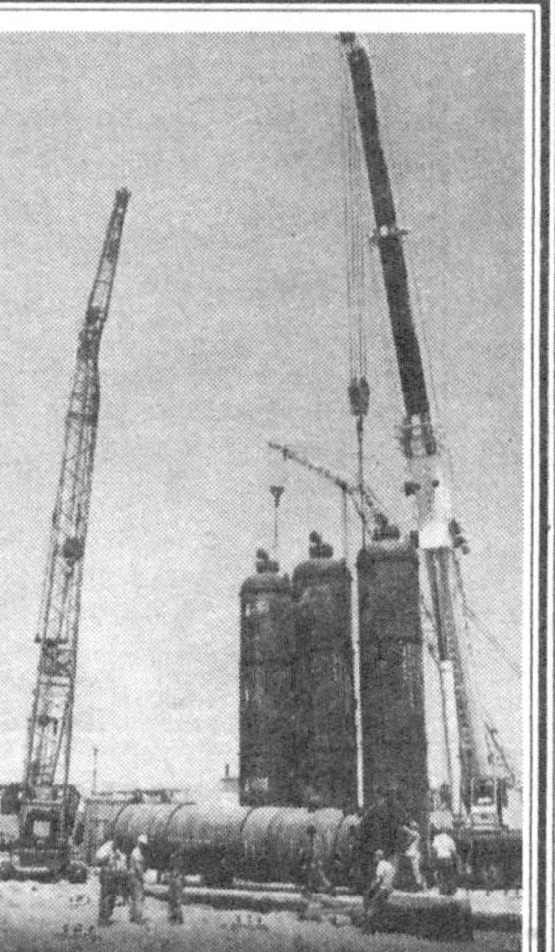
По всему объекту ведут монтажные работы строители Представительства № 9 АОТ «Мубарекнефтегазстрой». Сборка аппаратов воздушного охлаждения газа ведется бригадой Ш. А. Абдуллаева, начальника участка В. М. Конорева (на снимке); монтаж аппаратов адсорберов серочистки газа.
