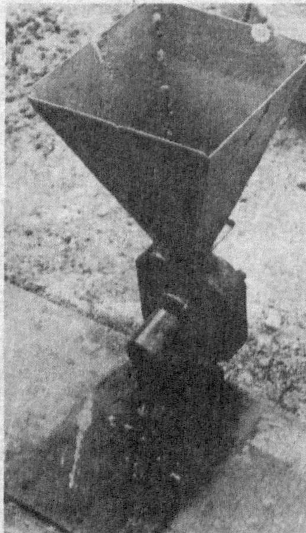
Микромельница ММ-50
