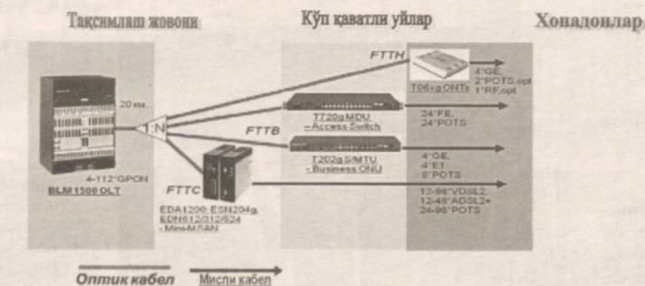
Оптик структура FTTx тармоғи қурилишлари куйидаги вариантлар асосида ташкил этилади.
