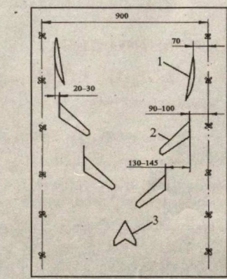
1-сферик диск; 2-пичоқ; 3-ўқёйсимон панжа. 2-расм. Қатор ораларида бегона ўтларни йўқотиш учун иш органларини жойлаштириш схемаси
