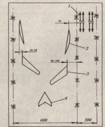
1-ротацион юлдузча; 2-сферик диск; 3-пичоқ; 4-ўқёйсимон панжа. 4-расм. Кўш қаторни экилган майдонларда бегона ўтларни йўқотиш учун иш органларини жойлаштириш схемаси
