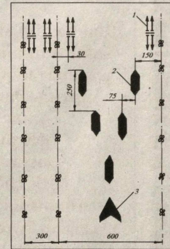
1-ротацион юлдузча; юмшаткич панжа; 3-ўқёйсимон панжа. 3-расм. Кўш қаторни майдонларга қатламлаб ишлов бериш учун иш органларини жойлаштириш схемаси
