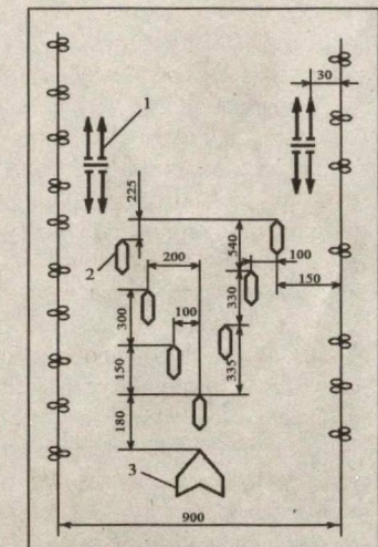
1-ротацион юлдузча; 2-юмшаткич панжа; 3-ўқёйсимон панжа. 1-расм. Қатор ораларида дастлабки юмшатиш учун иш органларини жойлаштириш схемаси
