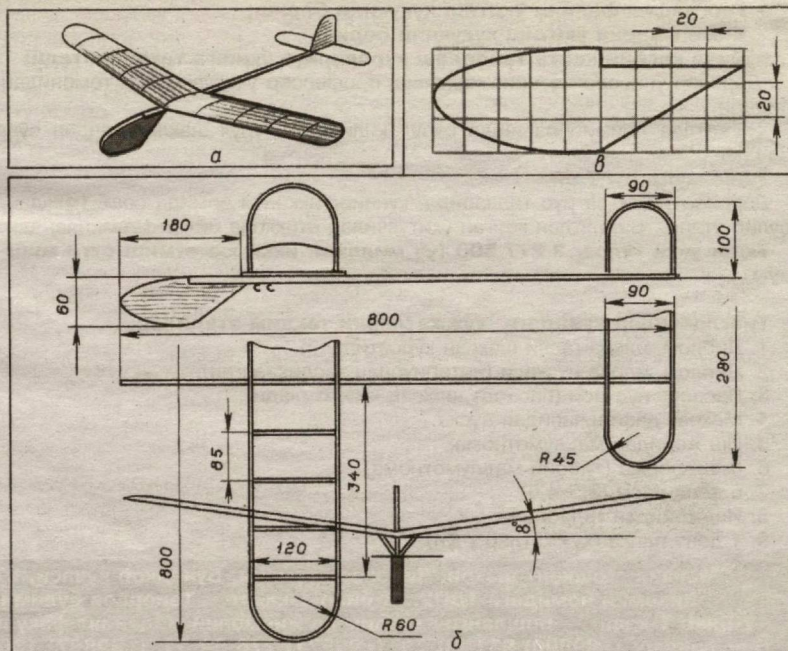
Расм. "Читтак" планери модели а — умумий кўриниши; б — чизмаси; в — юк шаблони
