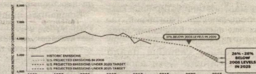
3-расм. АҚШнинг 2020 ва 2025 йилларда CO_2 газини ҳавога чиқаришини камайтириш бўйича режаси.
