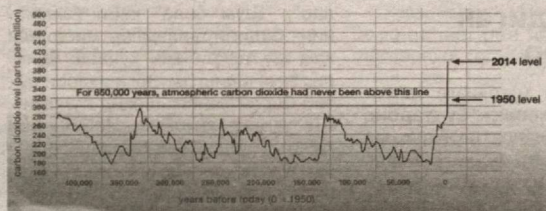
1-расм. Атмосферада CO_2 газининг ўзгариш даражаси.
