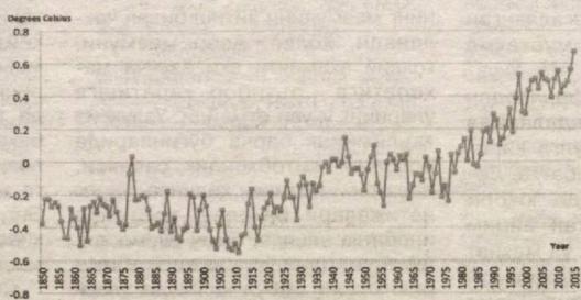
2-расм. 1850—2015 йилларда ер шариде ўртача ҳароратининг ўзгариши.
