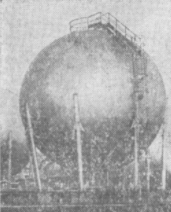
ТАТАРСКАЯ АССР. Нижнекамский нефтехимический комбинат — предприятие с полным циклом переработки нефти — готовит сырье для девяти пятилетки. Оно увеличило выпуск продукции почти в десять раз. На комбинате выпускают самые дешевые в стране синтетические каучуки, некоторые из них по своим достоинствам превосходят натуральные. На снимке: шаровые емкости со сжиженным газом. Фото Е. ЛОГВИНОВА.
