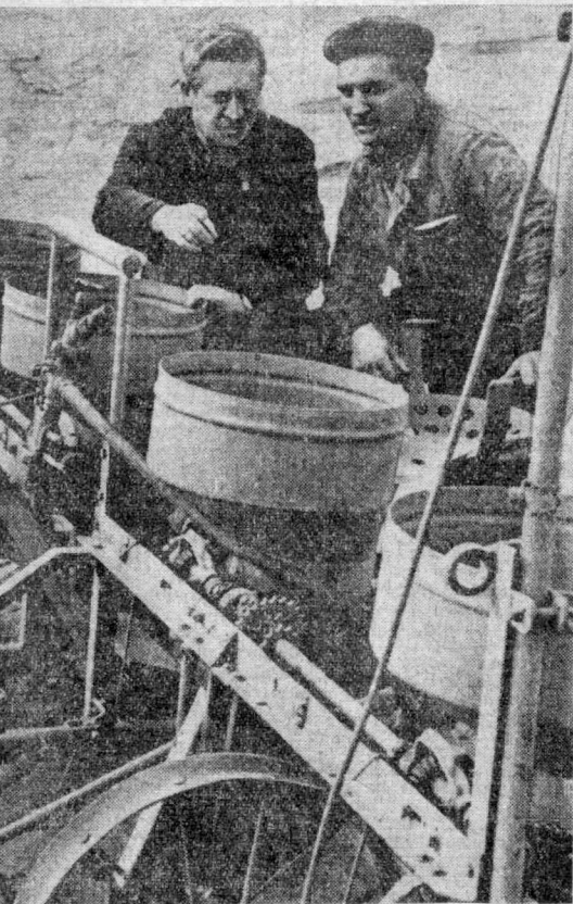
Коллектив завода «Узбексельмаш» осваивает новую четырехрядную хлопковую частотно-регулируемую сеялку «СХ-4А-1». На снимке: начальник мехоборудования цеха Л. И. Лещинер (слева) и бригадир слесарей-сборщиков Д. В. Кудренко осматривают новую сеялку.
