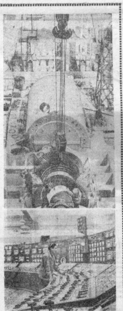
На Ташкентской ГРЭС горячие дни ударными темпами ведется монтаж шестого энергоблока. Он должен вступить в строй в конце нынешнего года. Коллектив строителей и монтажников работает дружно, чтобы уложиться в график. На снимке: монтаж турбины шестого энергоблока; у цеха управления одного из работающих энергоблоков.
