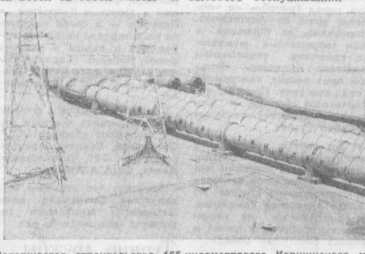
Завершается строительство 165-километрового Каршинского магистрального канала с шестью уникальными насосными станциями. В перспективе в Каршинской степи будет освоено свыше 900 тысяч гектаров засушливых земель. На снимке: одна из шести строящихся насосных станций.
