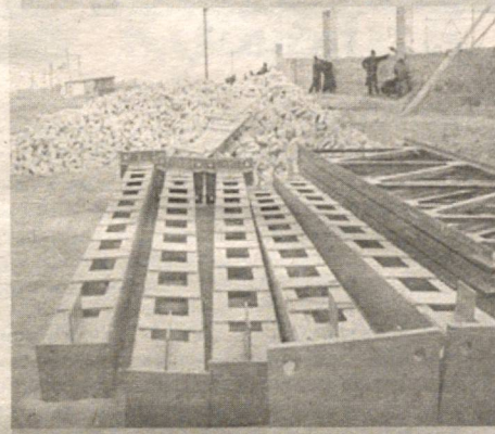
2009 йил декабр. Металл конструкциялар ўрнатилди бошланди.
