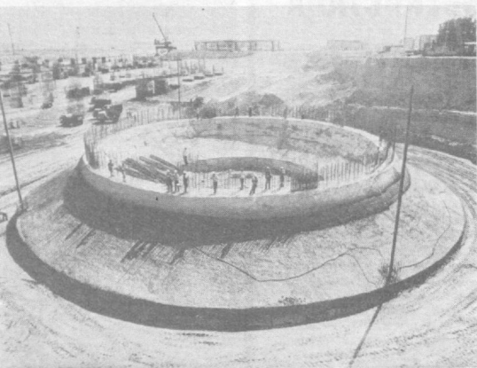
КАШКАДАРЬНСКАЯ ОБЛАСТЬ. Точно в срок завершил монтаж основания для дымовой трубы Талимарджанской ГРЭС инженер треста «Талимарджангострой» Сергей Щукин; готовый фундамент дымовой трубы Талимарджанской ГРЭС. Фото Ш. ШАРАПОВА (УЗТА).
