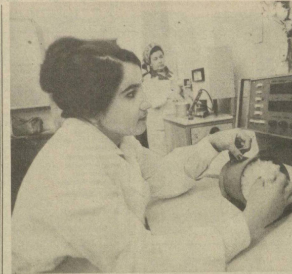
Новый прибор — анализатор сортности хлопца-сырца (АСХ-1) — используется в лаборатории Бектемирского опытного хлопкозавода Центрального научно-исследовательского института хлопководства УзССР. Через небольшое количество хлопца — до 150 граммов — под давлением пропускает воздух, и на табло фиксируется результат анализа: влажность, зорность. Весь процесс занимает считанные минуты. На снимке заведующий лабораторией С. Нуриллаева за работой с новым прибором. Фото УЗТАГ.
