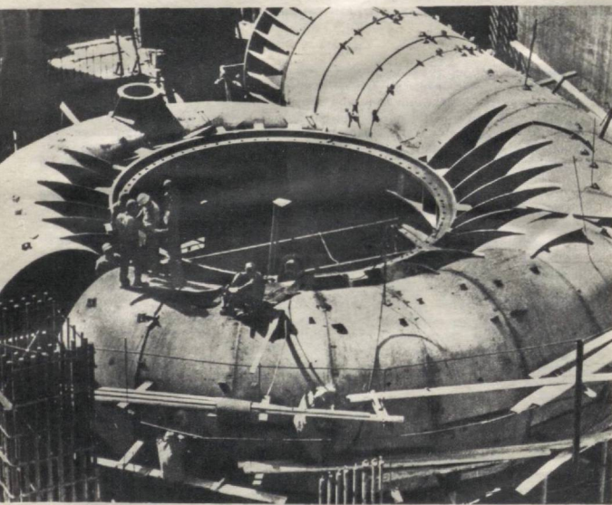
Тожикистоннинг сув ва нур ҳақидаги асрий орузи рўёбга чиқмоқда. Пулисангин қишлоғи яқинида қудратли Вахш дарёси ийовланиб, бу ерда Норақ ГЭСининг агрегатлари монтаж қилинмоқда.
