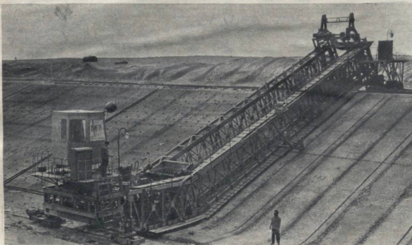
Қарши машина канали ўзанига бетон поёндоз тўшалоқда.
