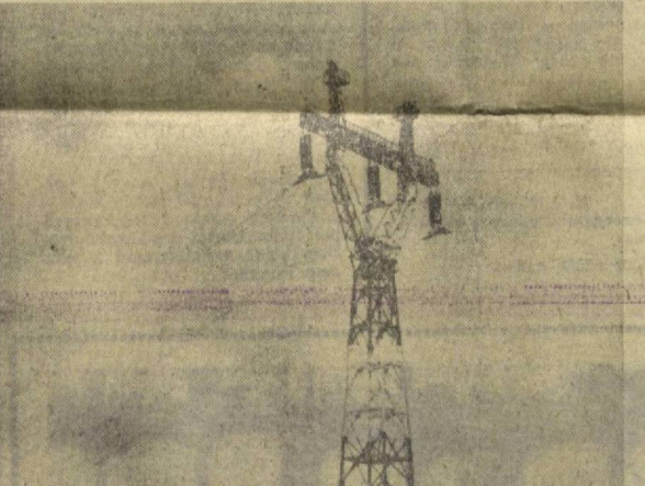
Вступила в строй линия электропередачи «Бочиноцы — Крайова». По ней Болгария через территорию Румынии будет получать ежегодно до 1 миллиарда кВт-часов электроэнергии из Советского Союза. Линия протяженностью 140 километров — плод сотрудничества СССР, РСР и НРБ.
